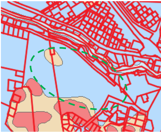
Kuva 5 - GTK:n yleispiirteinen Maaperäkartta, luettu 7.6.2022, (sininen= savi, vaalean ruskea= hiekkamoreeni, punainen=kallioma), kiinteistörajat MML 6/2022
