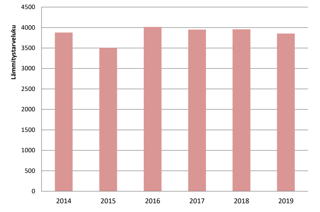
Kuva 4. Loimaan lämmitystarveluvut vuosina 2014–2019.
